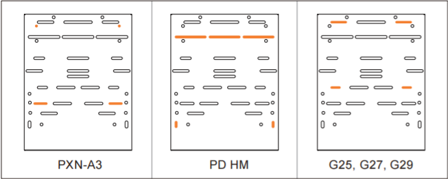
Lochdiagramm der Pedalplatte/ Kompatible Produkte (*teilweise)
