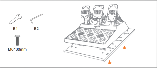
脚踏板孔位示意/兼容产品(*部分)
