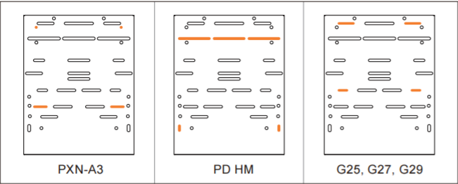
Schéma des trous de la plaque des pédales/ Produits compatibles (*partiels)
