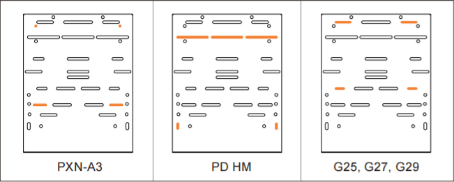
Diagrama de agujeros de la placa de pedales/ Productos compatibles (*parciales)
